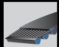
POLY CHAIN™ GT™ CARBON™
